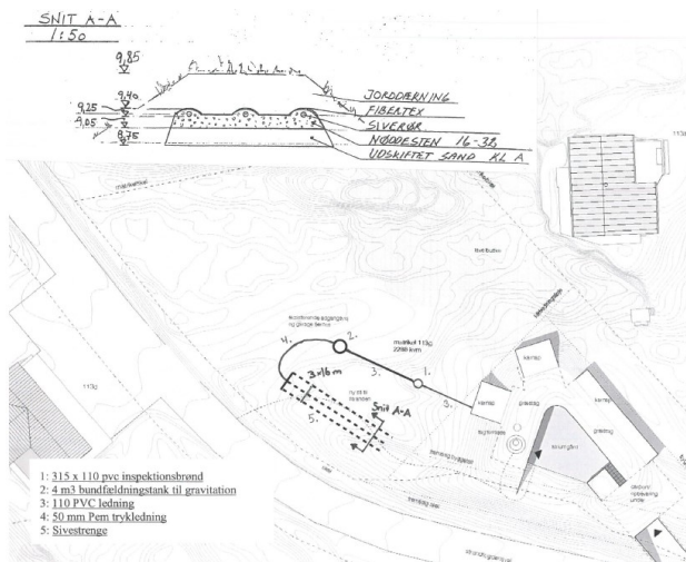
Nedsivningsanlæg med mile i forbindelse med jordvarme
