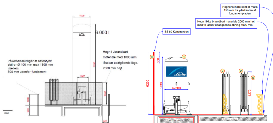
Fig. 3. Tegning over den eksisterende oxygentank (venstre) og den ansøgte oxygentank (højre).
