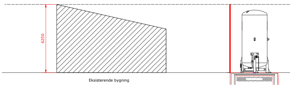
Fig. 4. Tegning over den ansøgte oxygentank i forhold til ejendommens bebyggelse.
