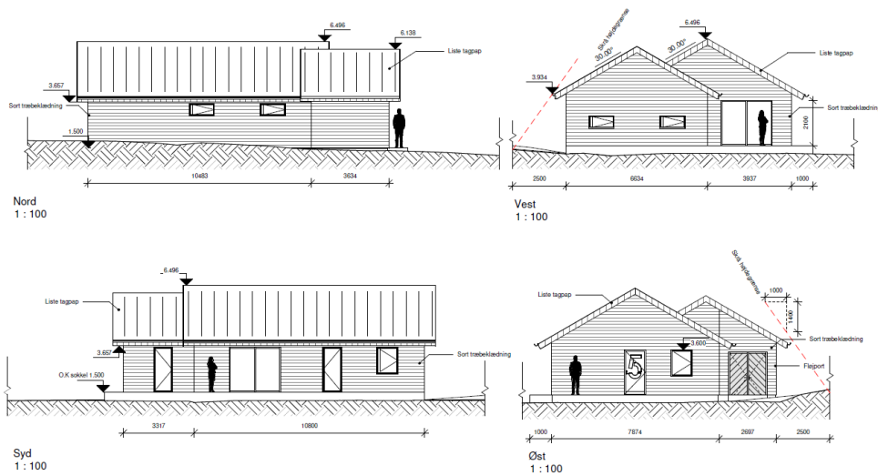
Figur 3: Tegning af det nye sommerhus
