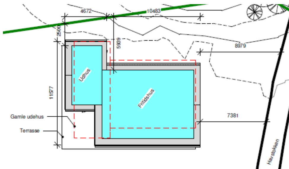
Figur 4: Situationsplan. Rød stiplede linje indikerer nuværende sommerhus
