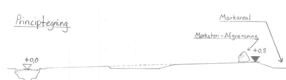
Fig. 5 – Princip-tegning af snit i ansøgt område til erstatningsnatur. Arealet nærmest åen terrænreguleres til nær kote 0,0 og vil have en næsten konstant hældning op til kote +0,8 m mod markarealet. Der tænkes udført mindre variationer i arealet for at opnå mulighed for lokale lavninger og variationer i landskabet (fra ansøgningen)
