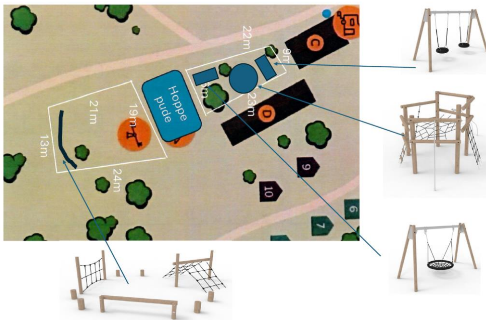
Fig. 2. Tilsendt fra ansøger. På figuren ses den ansøgte placering af legeredskaberne.
