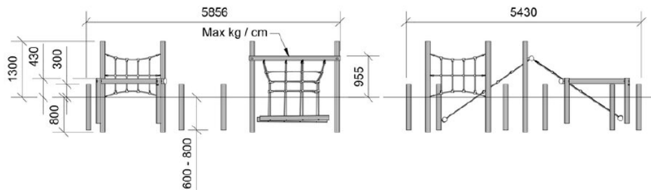
Fig. 6. Tilsendt fra ansøger. På figuren ses en illustration af den ansøgte forhindringsbane. På figuren ses målene på legereskabet.
