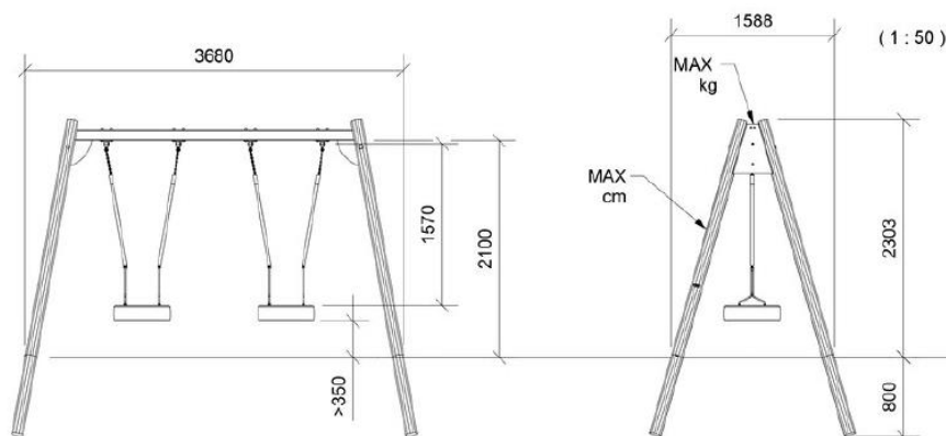
Fig. 4. Tilsendt fra ansøger. På figuren ses en illustration af det ansøgte gyngestativ med to sæder. På figuren ses målene på legereskabet.
