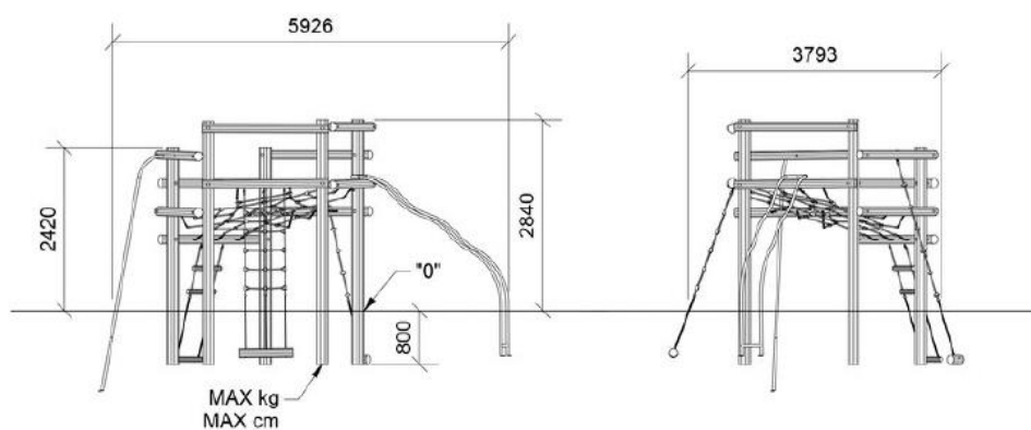
Fig. 5. Tilsendt fra ansøger. På figuren ses en illustration af det ansøgte klatrestativ. På figuren ses målene på legereskabet.
