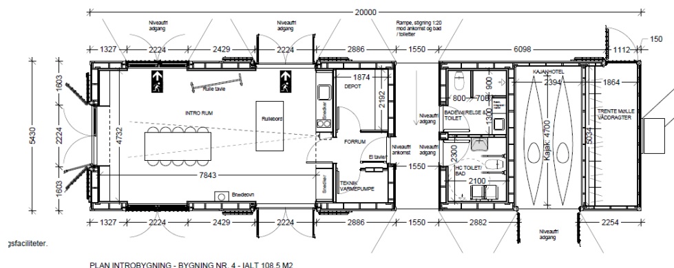
Grundplan bygning 4. Fremtidige forhold.
