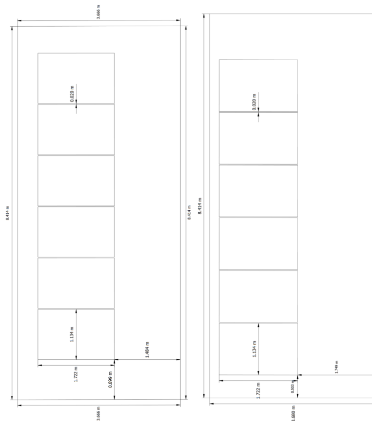
Fig. 3. Illustration indsendt af ansøger som viser mål på solcellepanel på hver tagflade.
