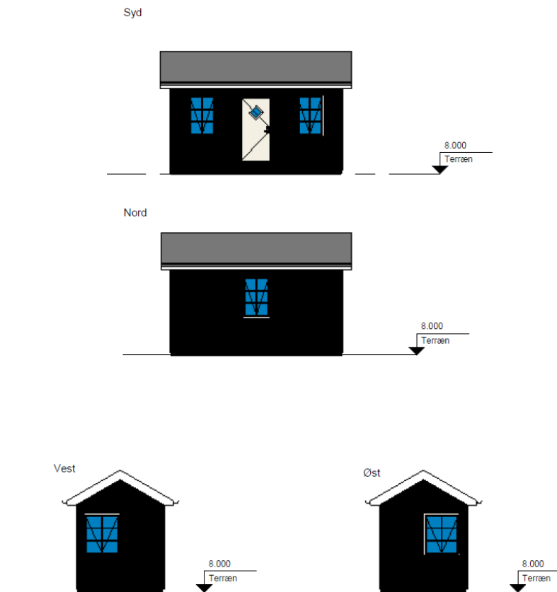
Fig. 4. Facadetegninger af det ansøgte anneks' fire facader.
