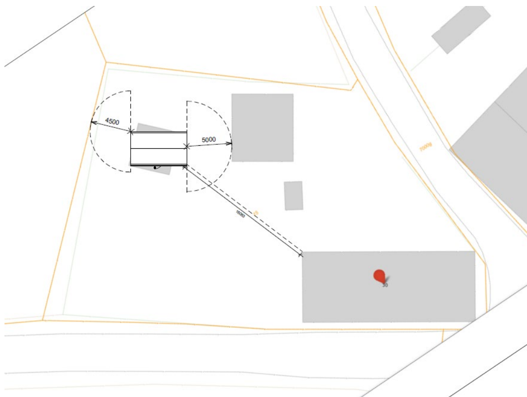
Fig. 3. Situationsplan over det ansøgte annek. Det grå indtegninger markerer de eksisterende bygninger. Det nye annek placeres på samme placering som det eksisterende.
