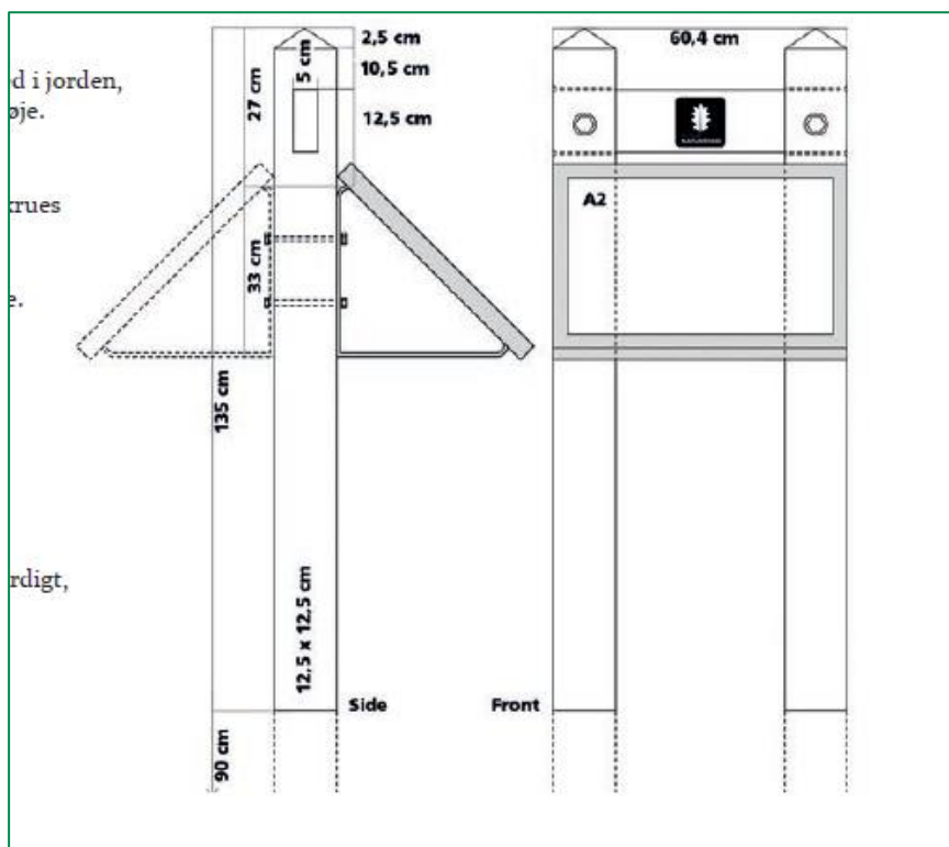
Fig. 4. Tilsendt af ansøger. Konstruktionstegning af skiltet.
