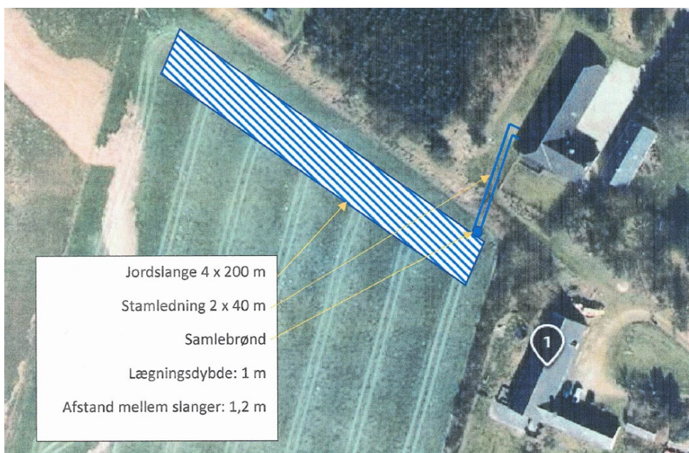
Situationsplan viser arealet, hvis der nedgraves slanger til jordvarme, samlebrønd og stamledning mellem ejendommen og brønden.
