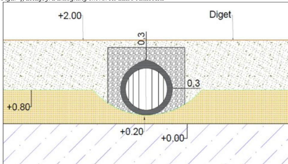
Figur 5, tegning fra ansøgning, der viser rørets udløb på kystsiden af diget
