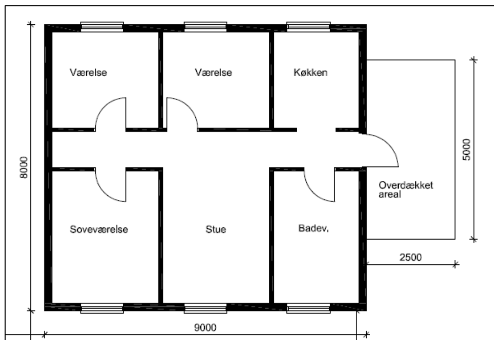
Plantegning for mandskabsvogn
