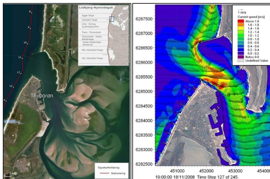
Figur A-1 Til venstre: sedimenttransport igennem Thyborøn Kanal medfører sedimentfaneaflejring i den vestlige del af Nissum Bredning, der gennemskæres af fire hovedløb i henholdsvis nordlig, østlig og sydlig retning (Rambøll, 2020). Til højre: øjebliksbillede af sydgående strøm langs den jyske vestkyst og indgående indadgående strøm i Thyborøn Kanal. Numerisk beregnet strømfelt (DHI, 2009).
