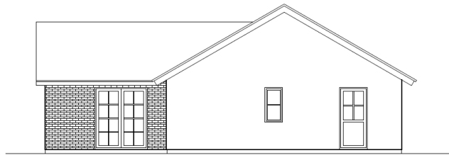
Øst facade
