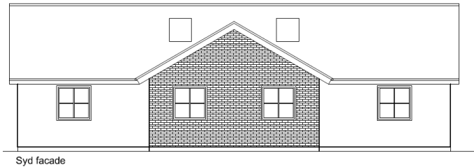
Syd facade
