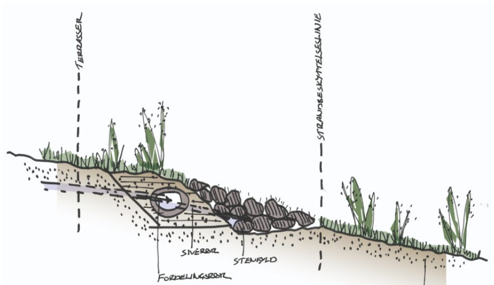
Principsnit for løsningen. Kystligger mod højre.
