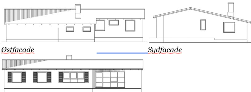
Eksisterende forhold
