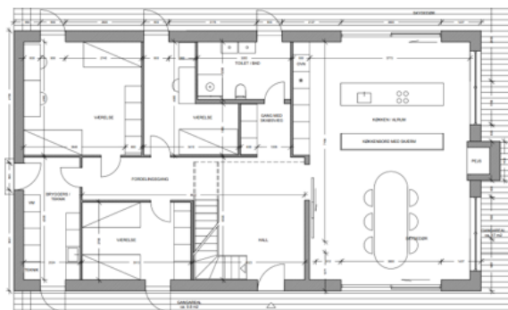
Stueplan
