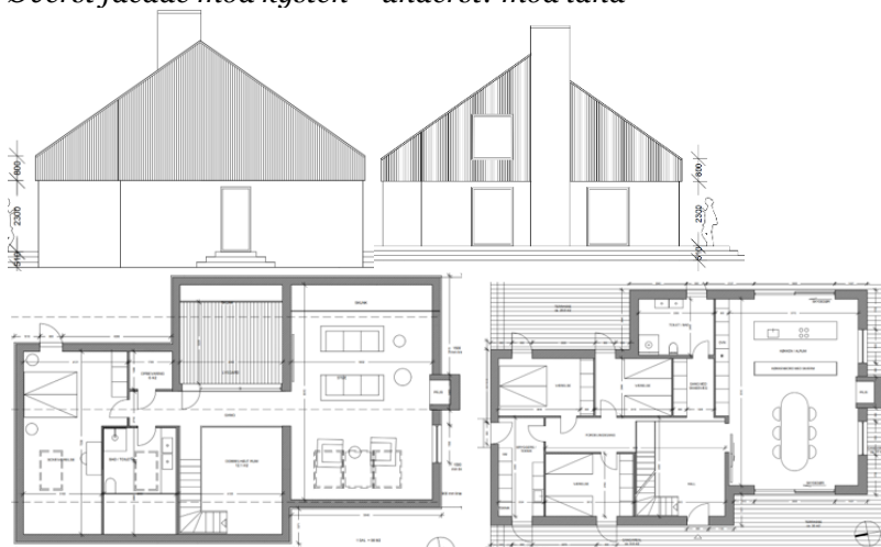
Grundplan stueplan
