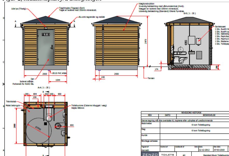
Figur 3, tegninger af toiletbygning, fra ansøgningen
