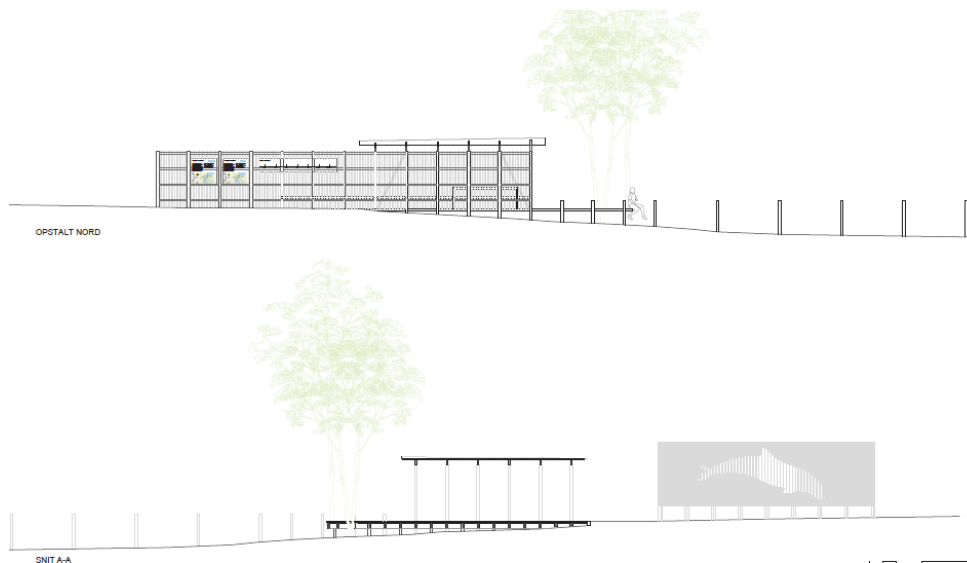
Figur 4, opstalt, fra ansøgningen
