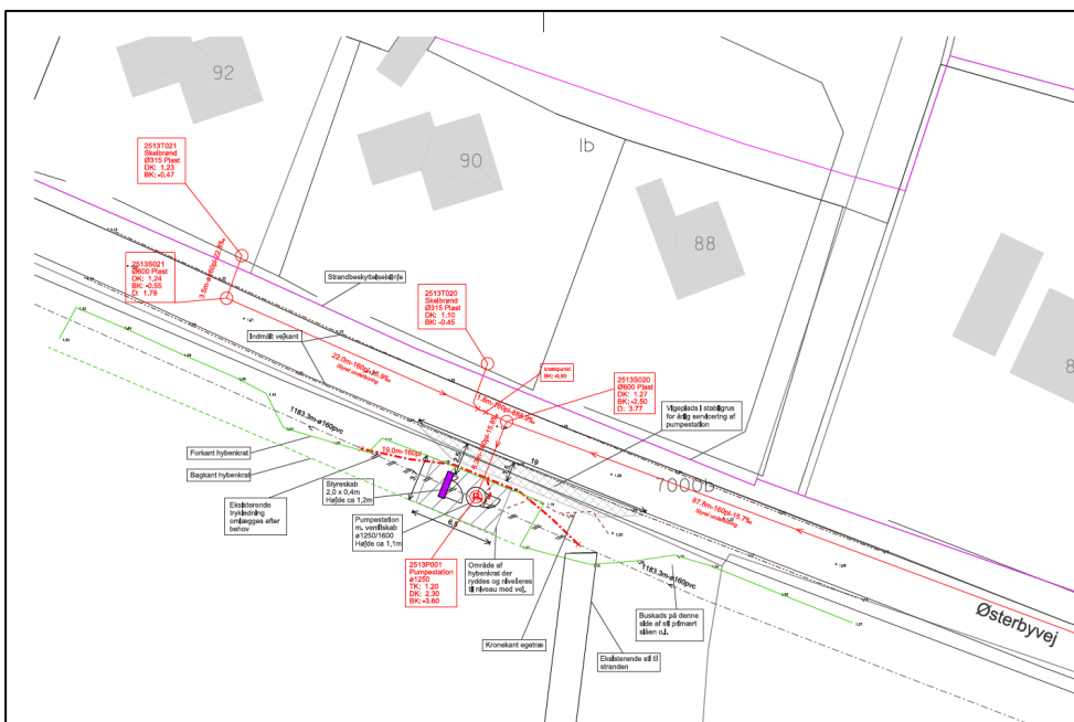
Fig.3. Tilsendt af ansøger. Byggetegning over anlægget. Pumpestationens placering er markeret med et rødt P. Styreskabets placering er markeret med lilla farve. Vigepladsen i stabilgrus er markeret med grå skravering.
