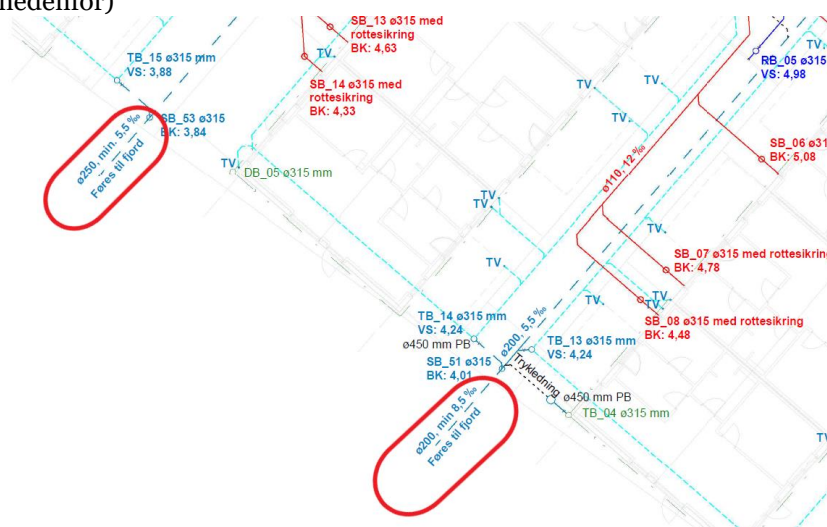
Fig. 4 viser en situationsplan over projektet. De to røde cirkler markerer hvor de to rørledninger til regnvand placeres. Indsat fra ansøgning.
