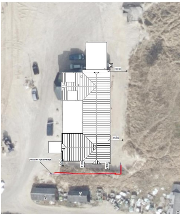
Stationen efter udvidelse – ny klitfodslinje vist rød
