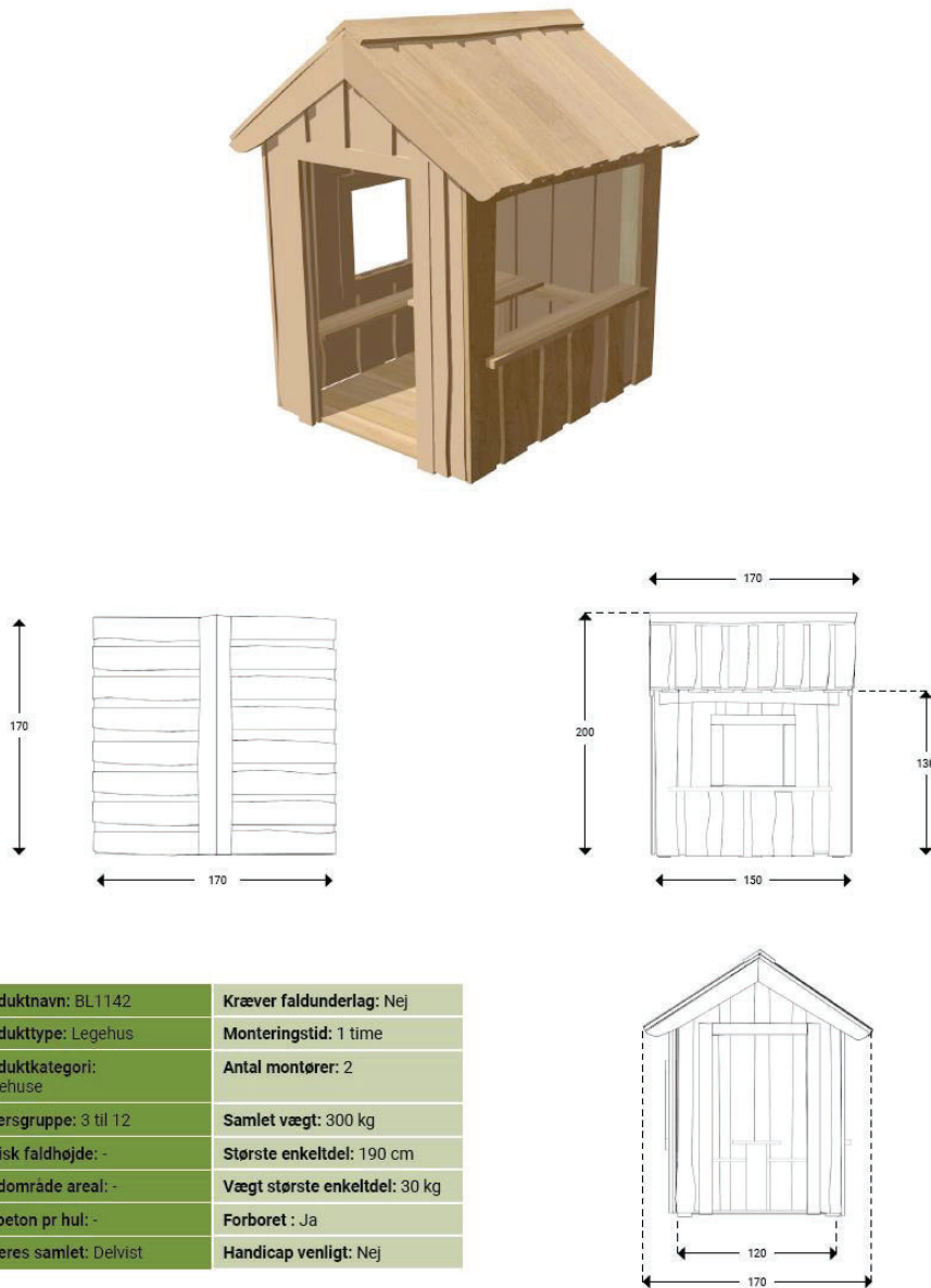
Fig. 10. Tilsendt fra ansøger. Datablad for legehus.
