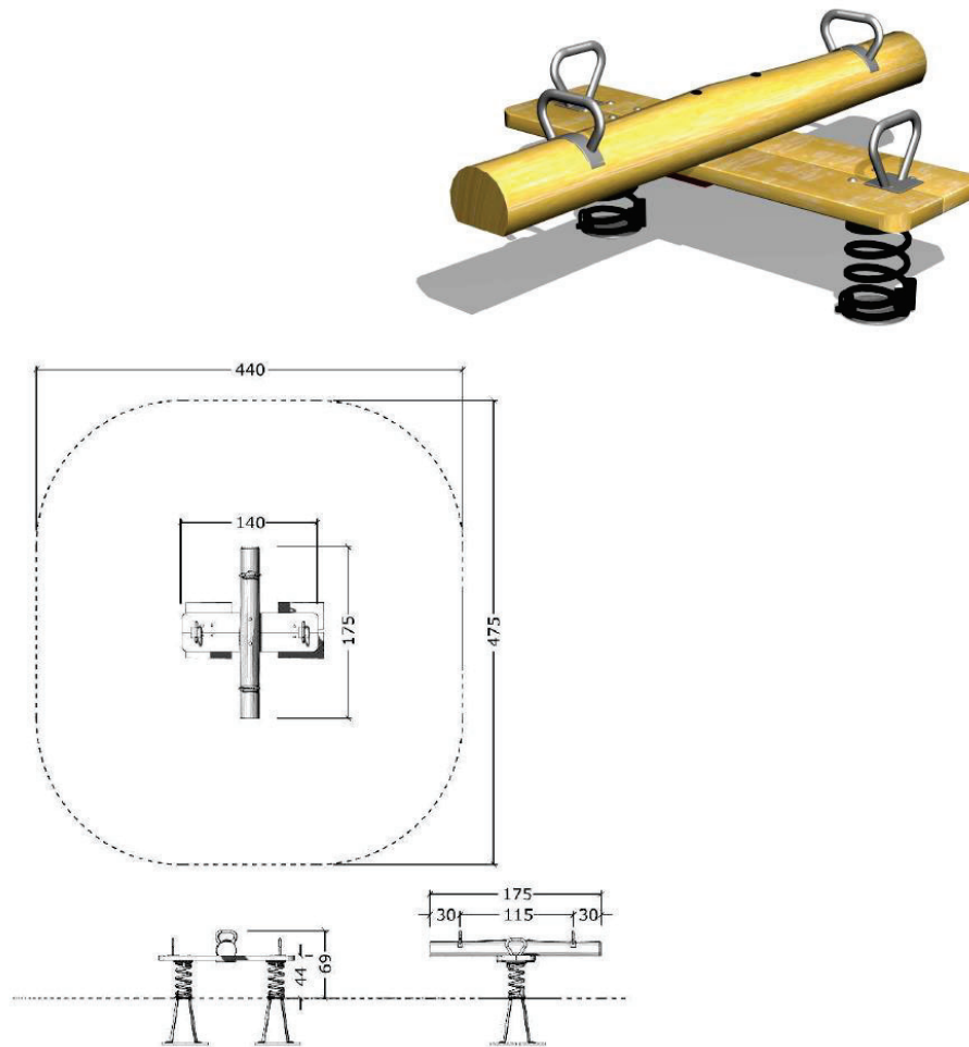
Fig. 6. Tilsendt fra ansøger. Datablad for vippe til fire personer.
