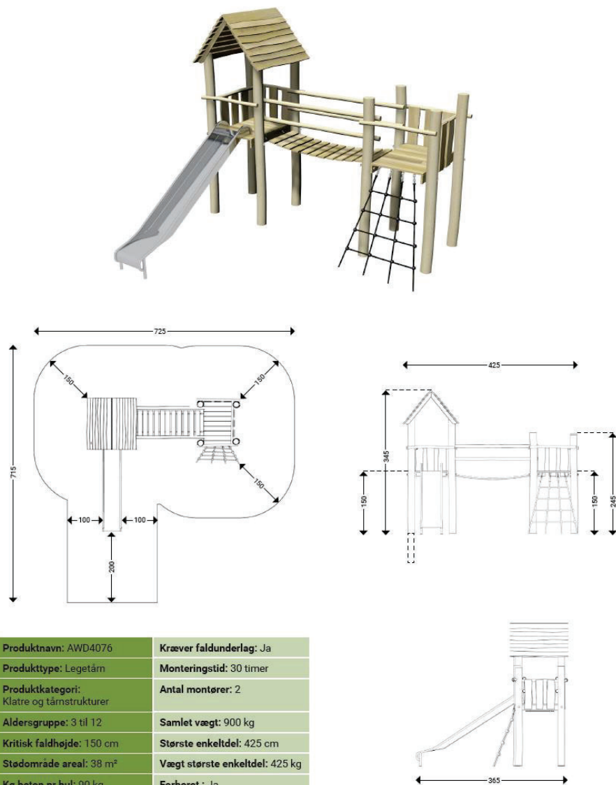
Fig. 7. Tilsendt fra ansøger. Datablad for legetårn.
