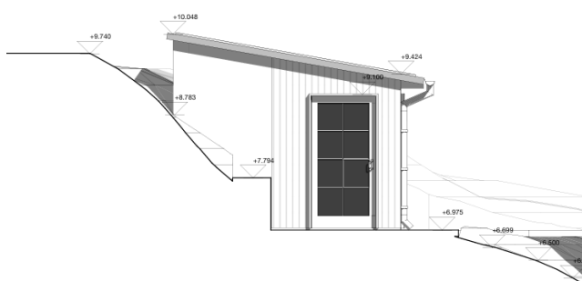
Opstalt – facade mod nord. Indsendt af ansøger.
