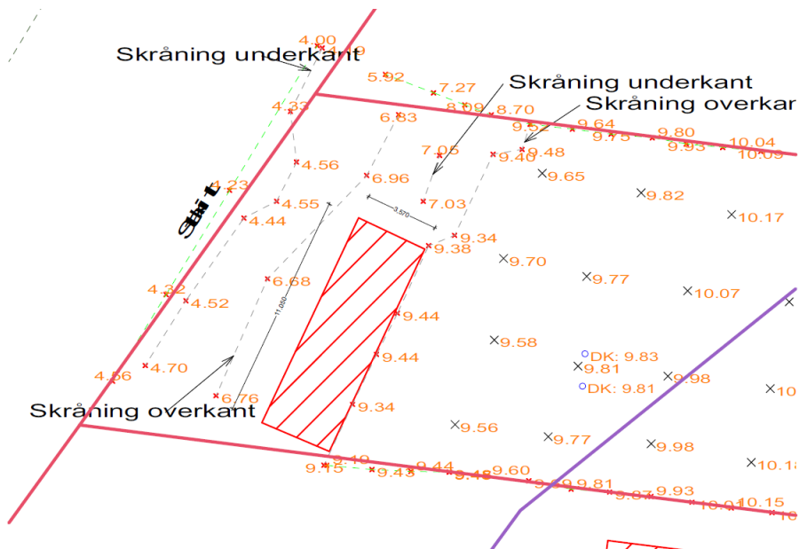
Landmålerens opmåling af eksisterende forhold. Indsendt af ansøger.
