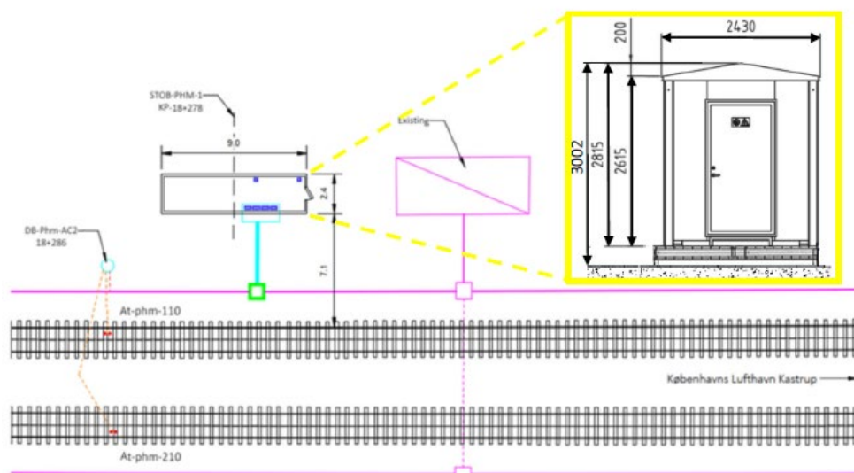
Fig. 4. Diagram over placering og strømforsyning ved jernbanen samt profil af hyttens vestlige ende med indgangsdør og mål i mm (fra ansøgningen)
