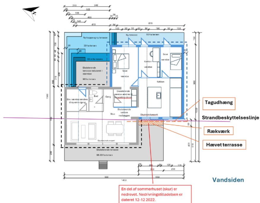
Fig. 2. Tilsendt fra ansøger. Plantegning med angivelse af det ansøgte og strandbeskyttelseslinjen.
