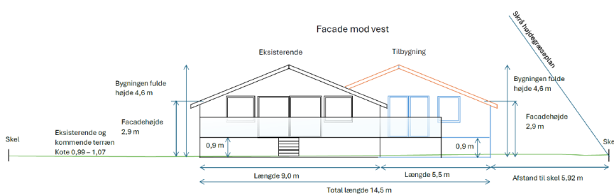
Fig. 4. Tilsendt fra ansøger. Facade mod vest. Sort angiver eksisterende forhold. Blå angiver tilbygning under opførsel og orange angiver det ansøgte tagudhæng.
