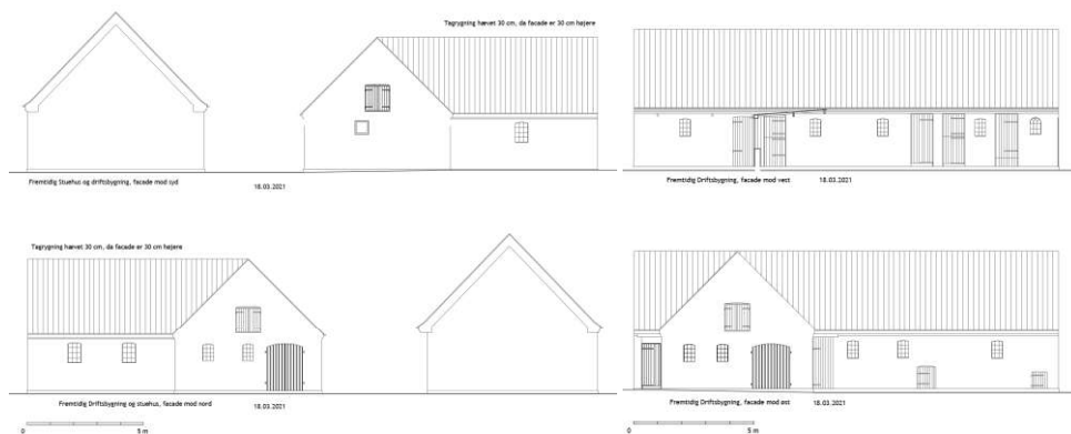
Fig. 3. Fremtidig bygning; tegninger af facader, indsendt af ansøger. Øverst/venstre=sydvendt, øverst/højre=vestvendt, nederst/venstre=nordvendt, nederst/højre=østvendt.
