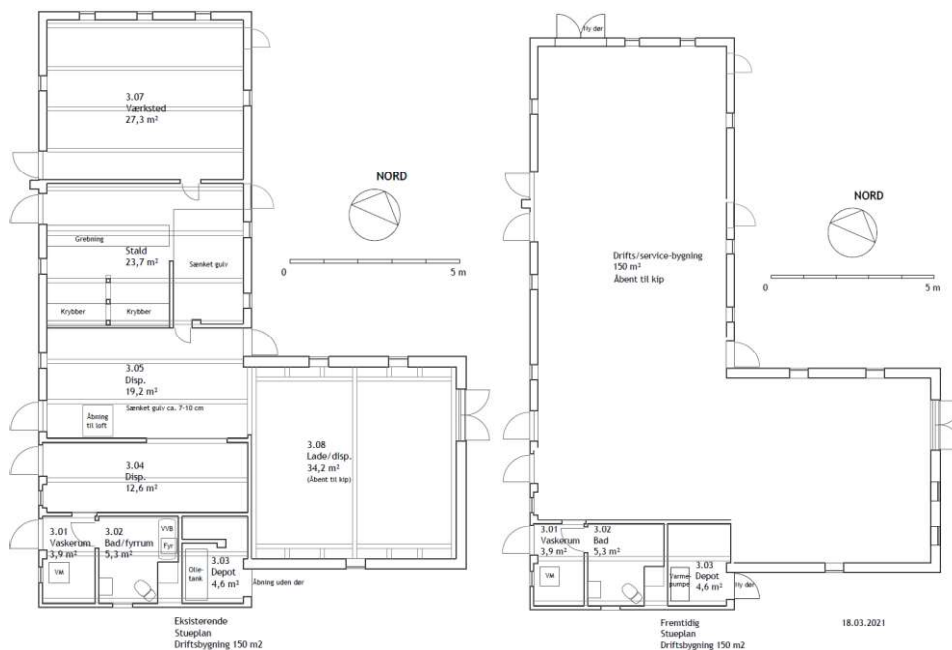
Fig. 4. Plantegninger indsendt af ansøger. Eksisterende bygning (venstre) og ansøgte bygning (højre).
