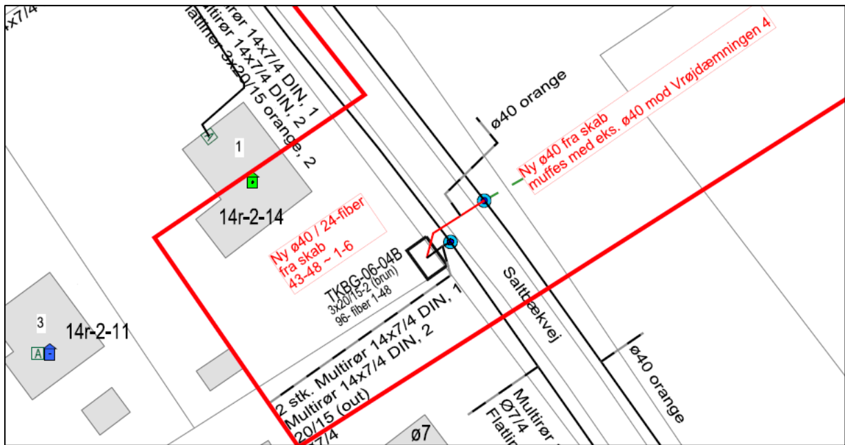
Detalje fra planen viser gravning ved Saltbækvej
