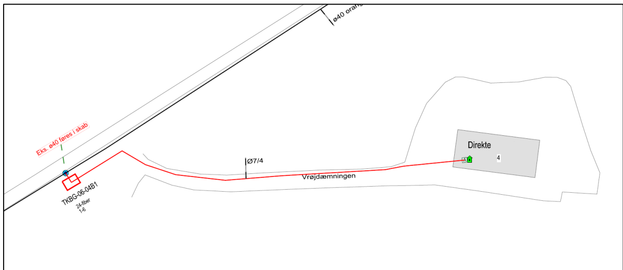
Detalje fra planen ved Vrøjdæmningen 4 viser placering af tekniskskab i vejsiden (vist med rød firkant) og det stykke, hvor der graves (rød linje).
