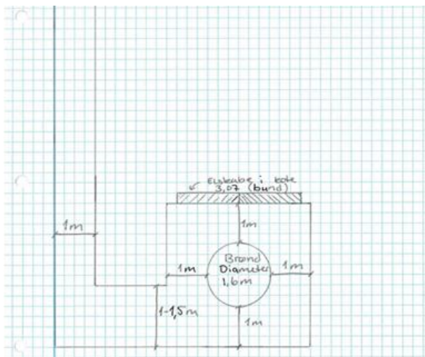
Fig. 7. Skitse fra ansøgningen. Viser dimensioner på afsats og platform, samt placeringen af de to nye skabe.
