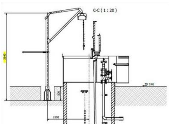
Fig. 10. Skitse fra ansøgningen. Viser en skitse over det nye hejseværk og brøndtoppen.
