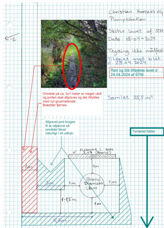
Fig. 11. Skitse fra ansøgning. Viser terrænændringer omkring afsats og platform ved pumpebrønden.
