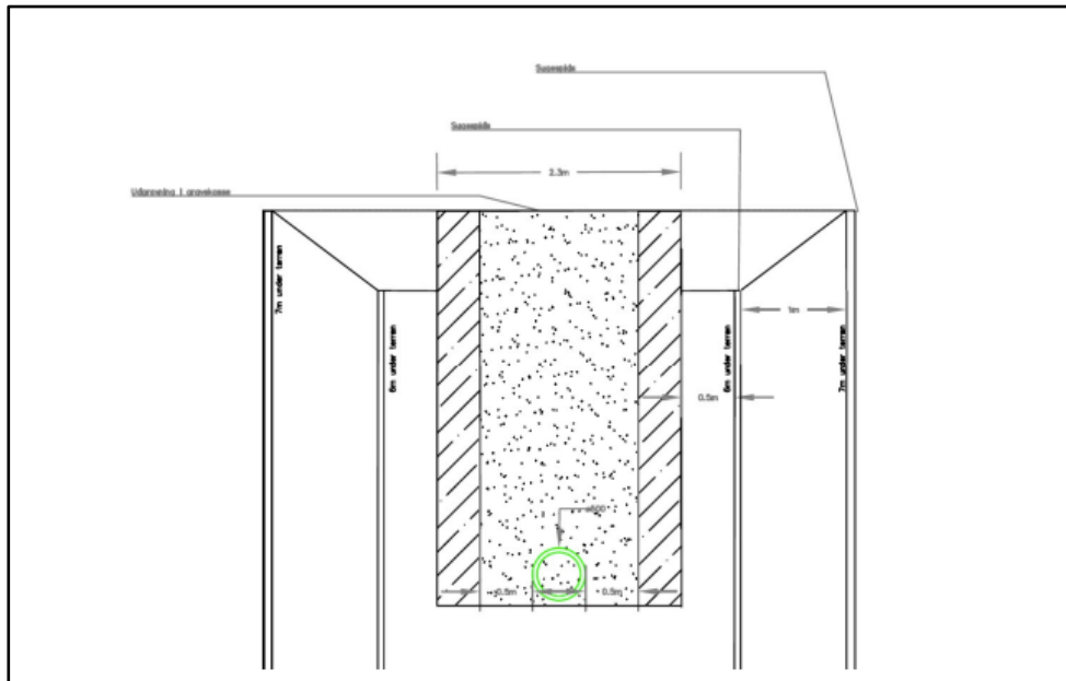
Fig 3, Tegning fra ansøgningen viser princip for en grave kasse og placering af dobbelt sugespidsanlæg til oppumpning af grundvand.
