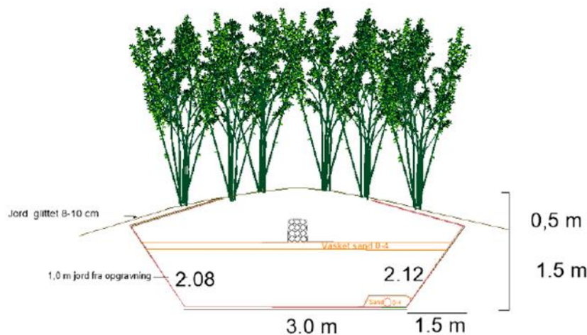
Fig. 5. Viser opbygningen af anlægget. Fra "dokumentation for størrelse og udseende af pilerenseanlæg". Fra ansøger.
