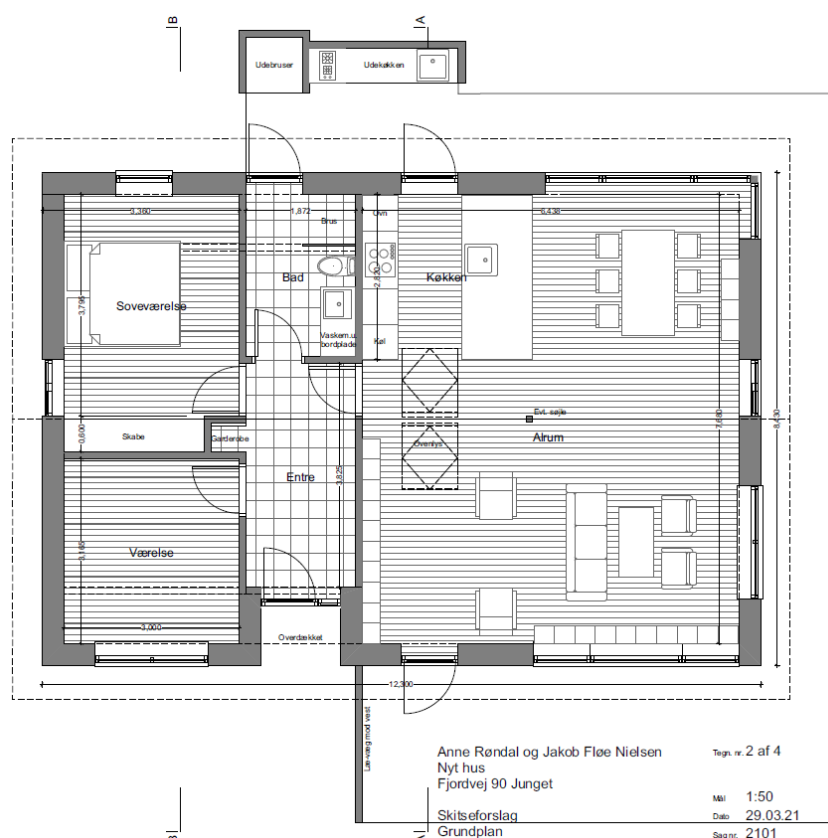
Figur 3: Grundplan for det nye stuehus. Søjlen i alrummet markerer placering af skorsten.
