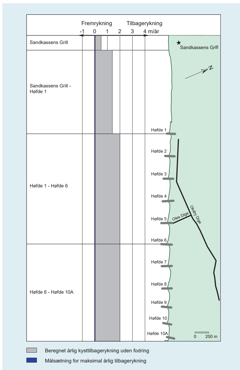
Figur 1 - Målsætning for kystudvikling i aftaleperioden 2027-2041.
