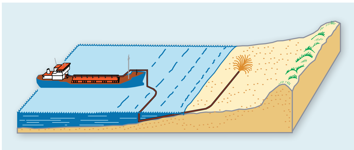
Figur 2 - Strandfodring med rørledning.
