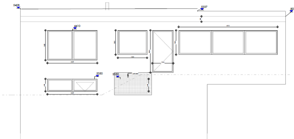
Fig. 3: Tegning vedhæftet ansøgningen. Facade syd.
