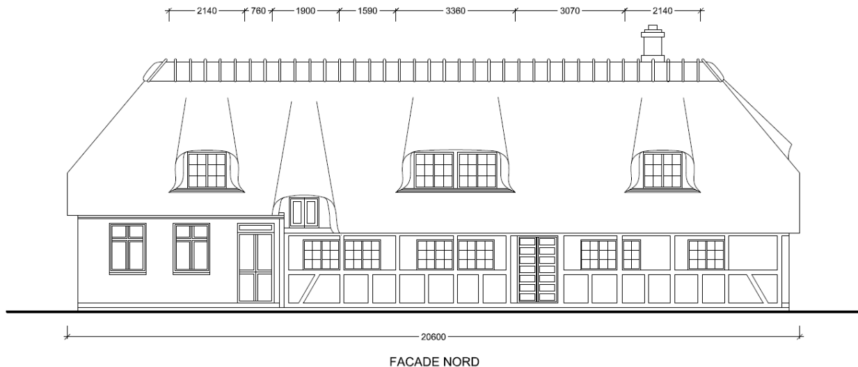
Fig. 7. Facadetegning af den fremtidige nordlige facade, indsendt af ansøger.
