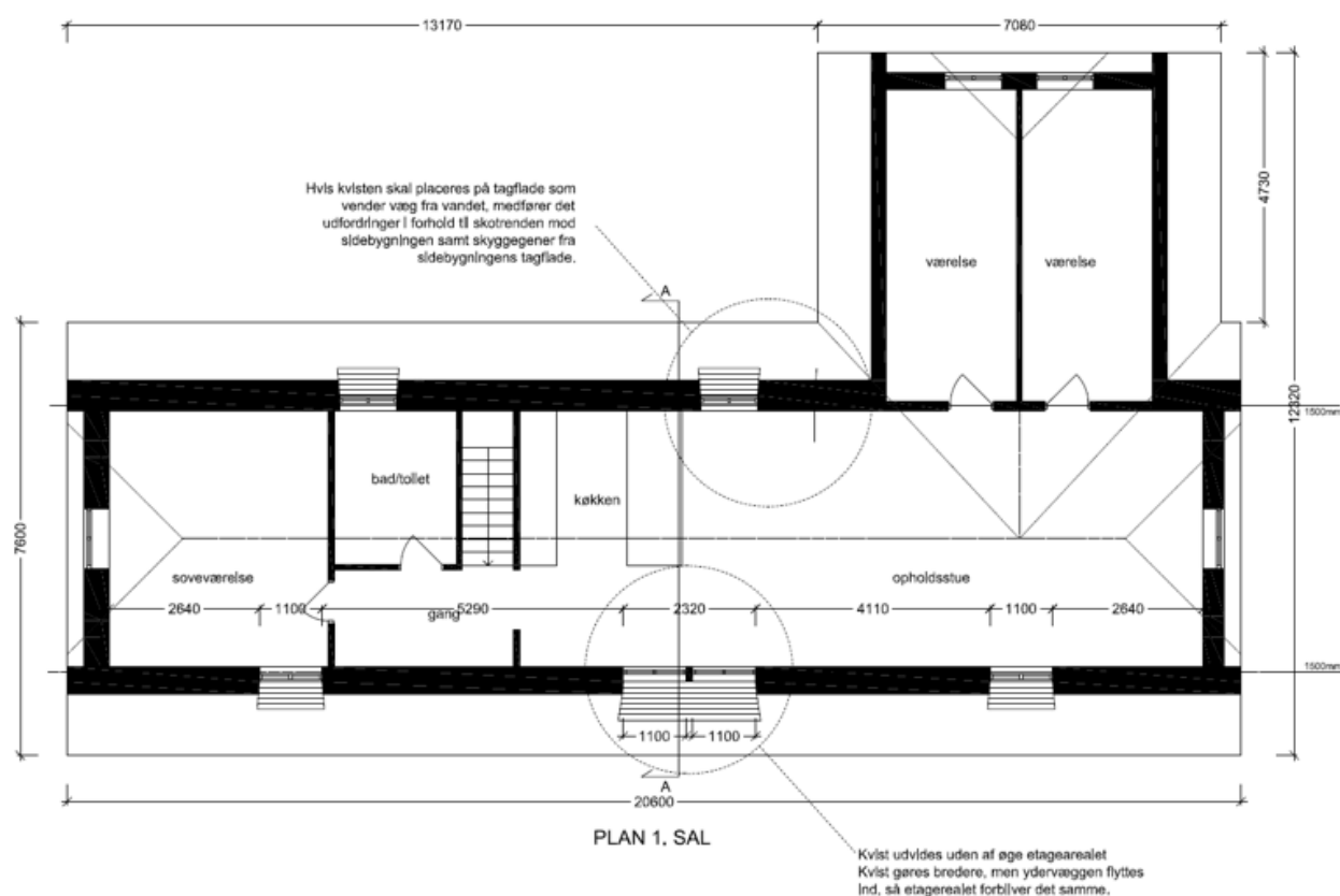
Fig. 5. Plantegning af de ønskede fremtidige forhold, indsendt af ansøger.
