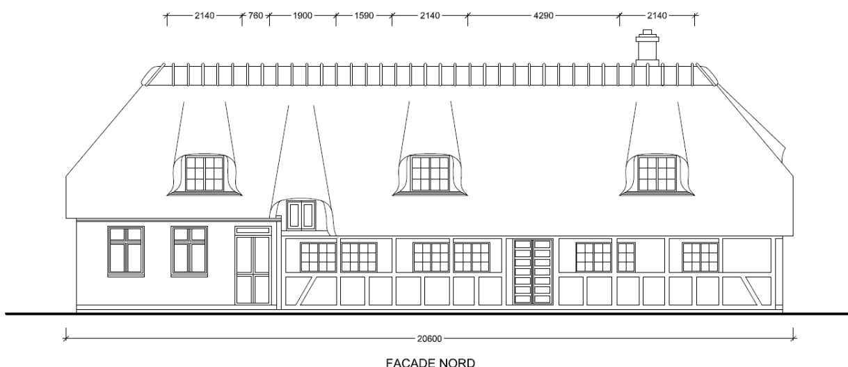
Fig. 6. Facadetegning af den nuværende nordlige facade, indsendt af ansøger.
