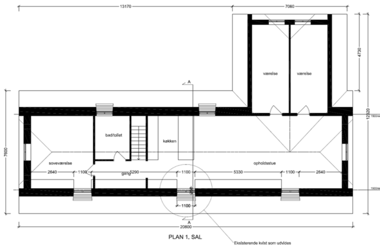
Fig. 4. Plantegning af de nuværende forhold, indsendt af ansøger.
