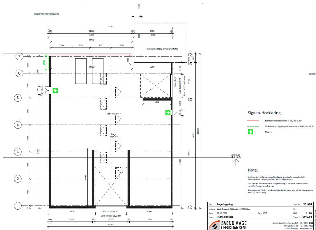
Teknisk tegning af udvidelsen af lagerhal, medsendt den oprindelige ansøgning
