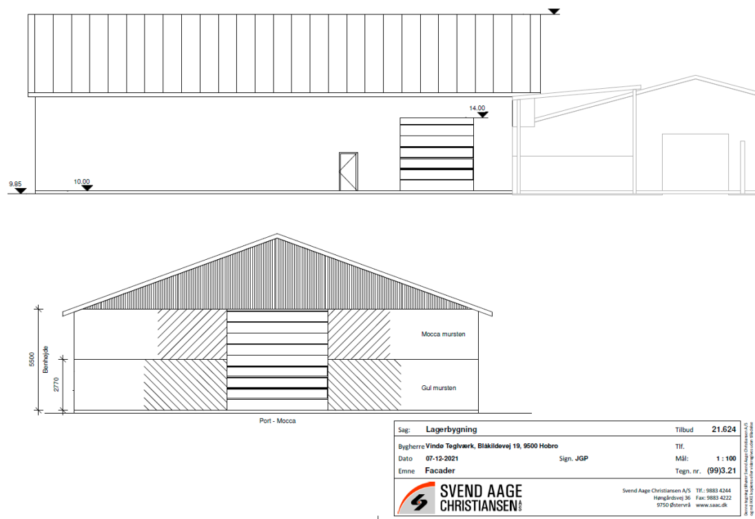
Facadetegning med dimensioner, medsendt den oprindelige ansøgning
