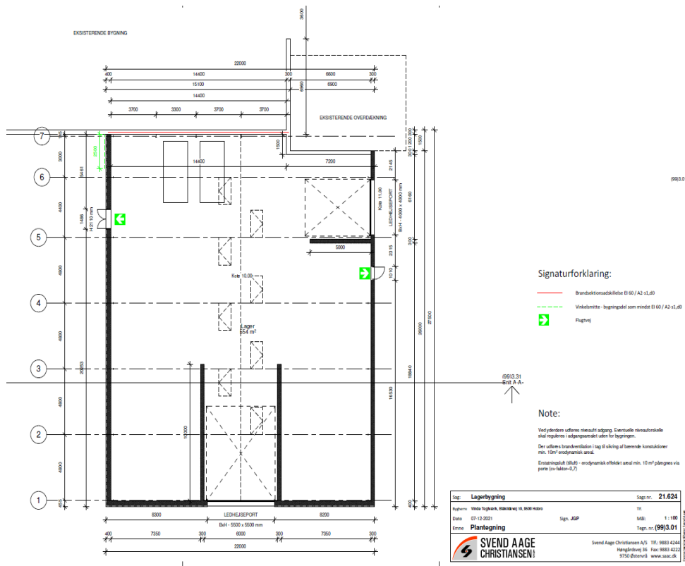
Fig. 4. Teknisk tegning af udvidelsen af lagerhal på 595 m 2 .
