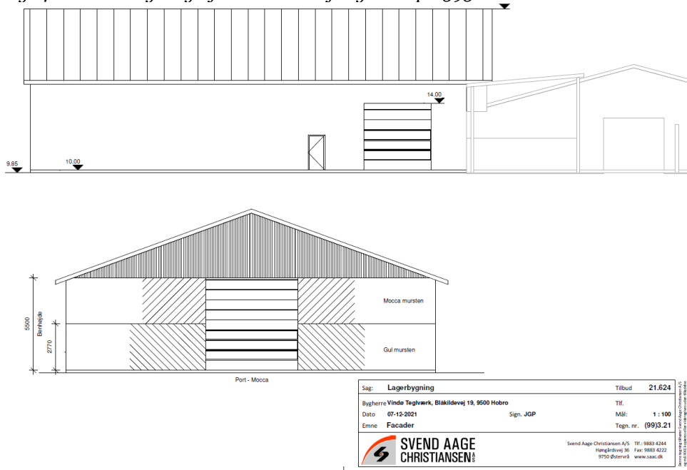
Fig. 4. Teknisk tegning af udvidelsen af lagerhal på 595 m 2 .
