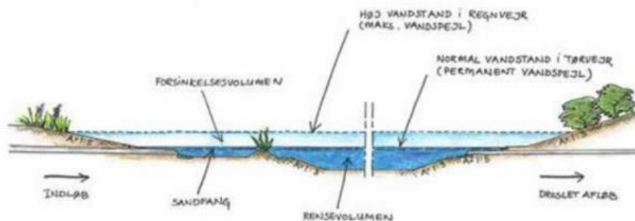
Principskitse for tværsnit i vådt bassin – figur fra §3 dispensationen.
