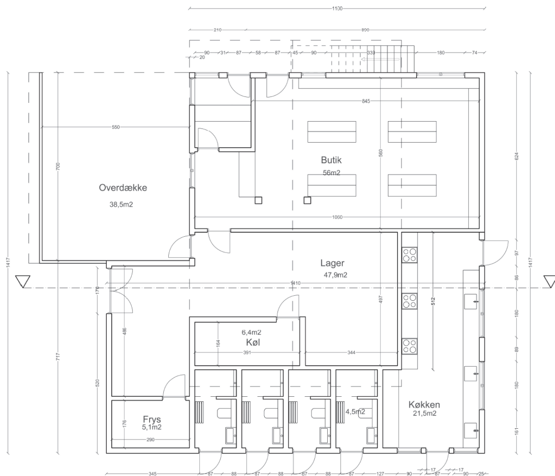
Fig. 13. Tilsendt fra ansøger. Den ansøgte plantegning af stueetagen.
