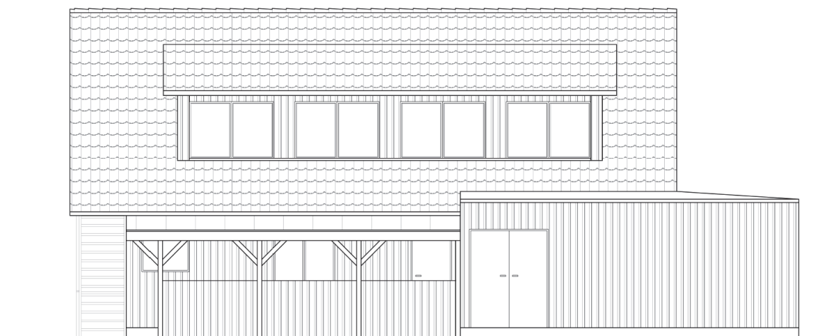
Fig. 11. Tilsendt fra ansøger. Den ansøgte vestvendte facade.
