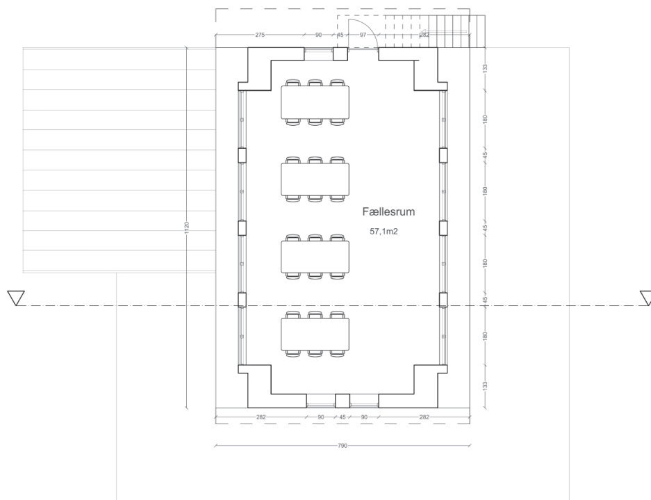
Fig. 15. Tilsendt fra ansøger. Den ansøgte plantegning af 1.sal.
