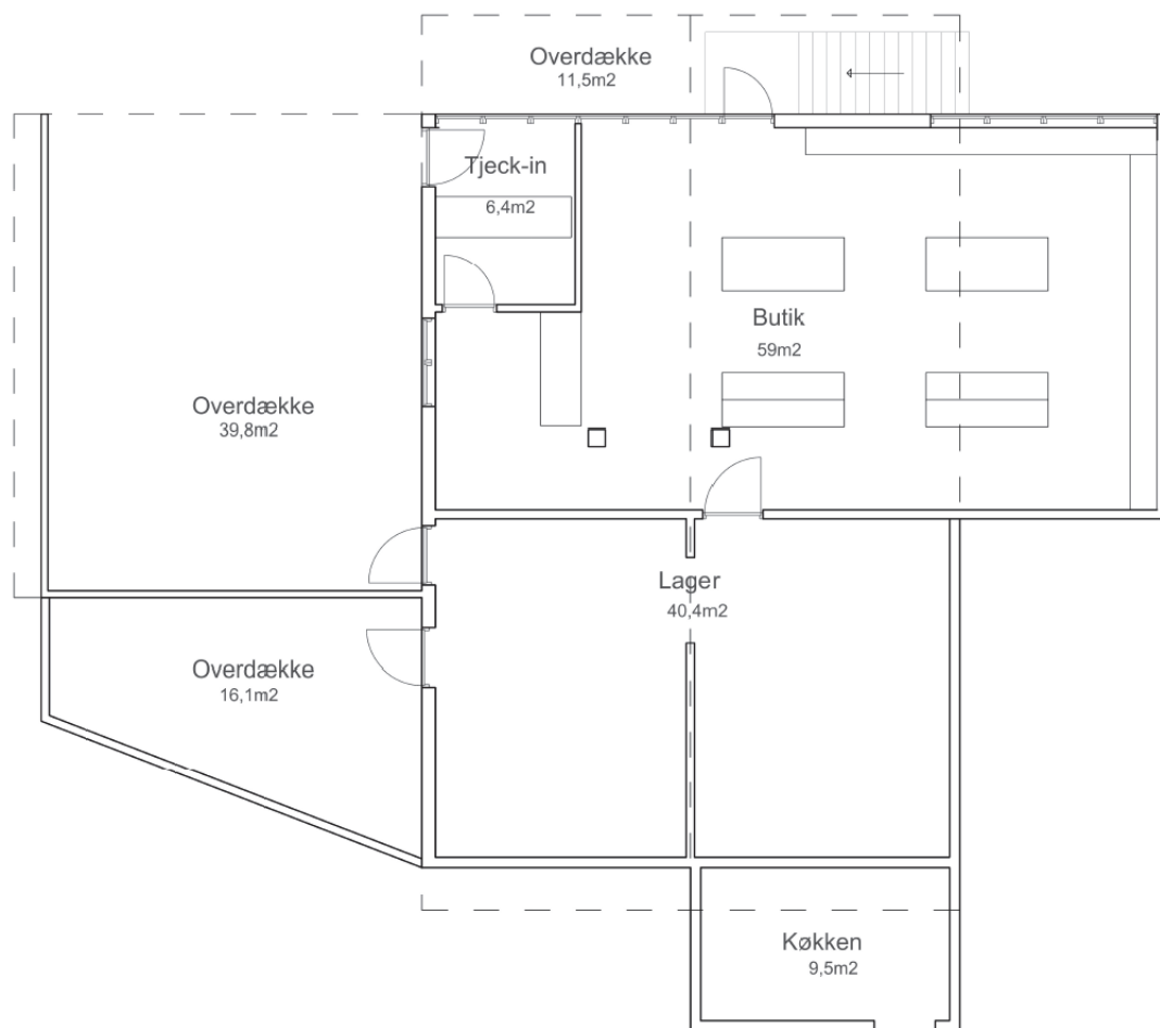
Fig. 12. Tilsendt fra ansøger. Den nuværende plantegning af stueetagen.
