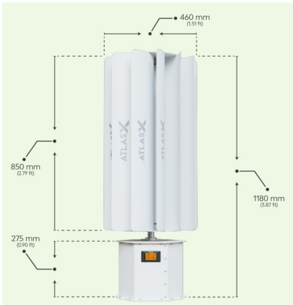
Tesup AtlasX vindturbine. Indsat fra produktblad på producentens hjemmeside.
