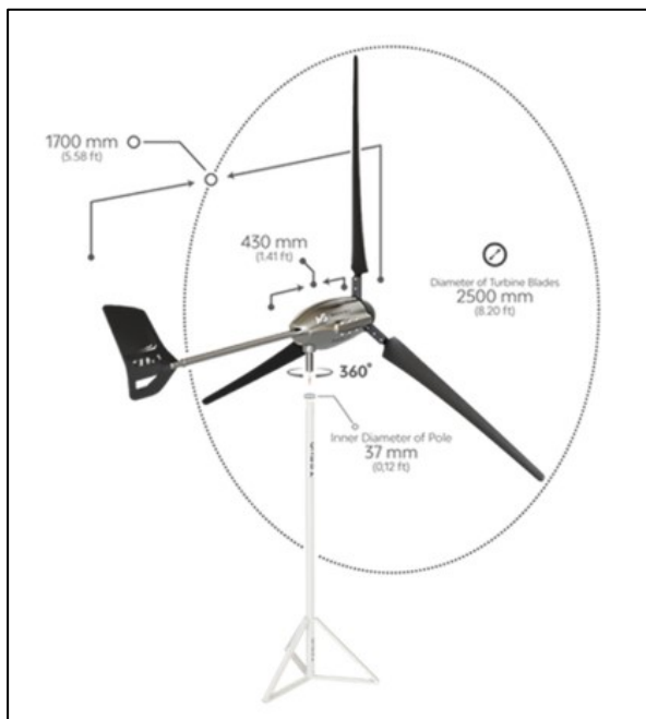
Tesup Magnum 5 vindmølle. Diameter på rotorblade er 2,5 meter. Indsat fra ansøgningsmaterialet.
