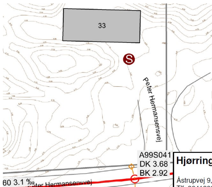
Fig. 2. Tilsendt fra ansøger. Den røde cirkel med et 'S' markerer placeringen af den eksisterende septiktank der fjernes. Den orange firkant nede ved vejen markerer det afproppede stik i ledningen på Peter Hermansensvej. 1 m inde på matriklen, ud fra denne, etableres den nye skelbrønd uden for klitfredningslinjen.
