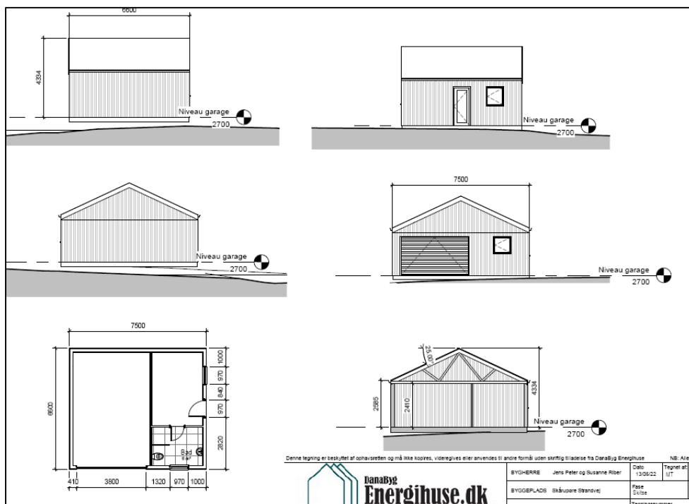
Tegninger af den nye bygning indeholdende garage/udhus.
