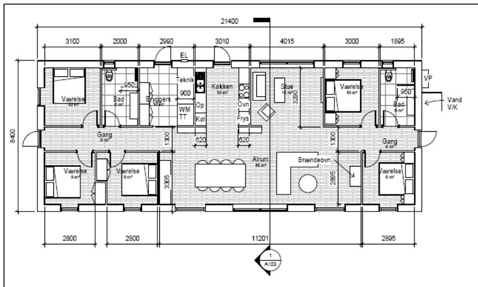
Grundplan for det nye sommerhus
