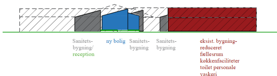
Principtegning af bygninger set fra øst. Skravering viser bygningsdele, der nedrives.
