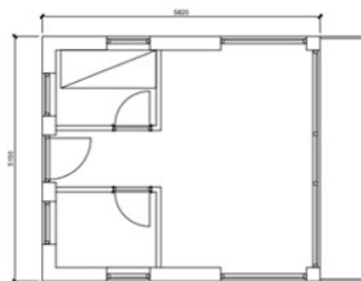
Plan 1:50 - 30m 2
