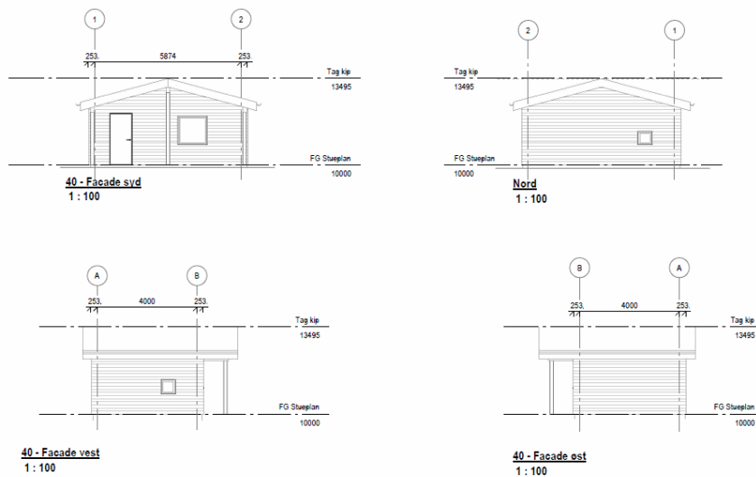
Figur 4, facadetegninger, fra ansøgningen
