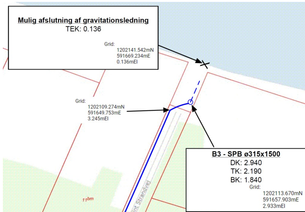
Figur 3. Detalje af planen ved udløbet og pumpestationen.
