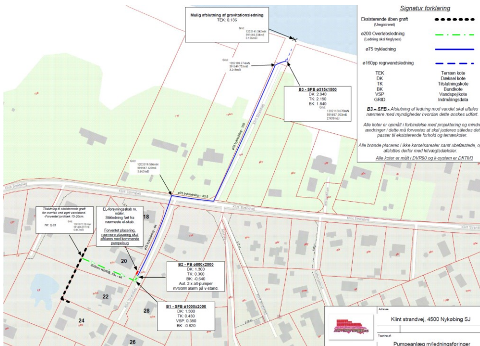
Figur 2. Tegning viser den projekterede ledningsføring fra grøften nederst til venstre på figuren til pumpestationen og havet øverst.
