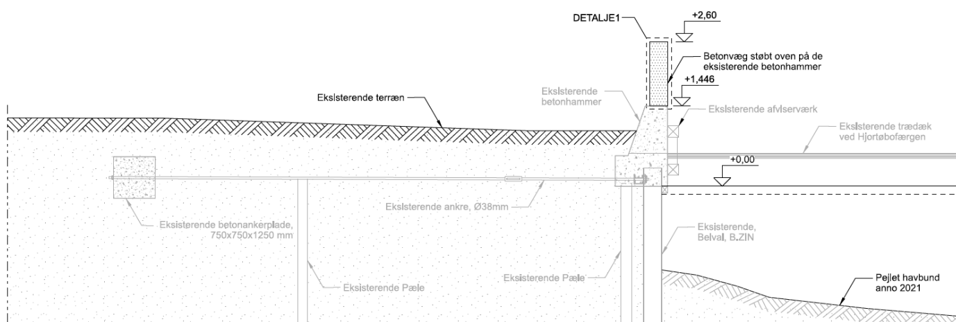
SNIT C3-C3, 1:50 Højvandssikring ved enden af Pakhuskajen
