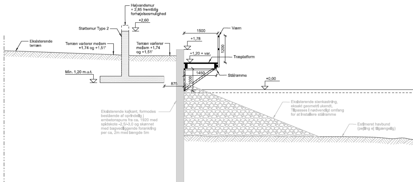
SNIT E3-E3, 1:50 Højvandssikring på Gasværkskaj
