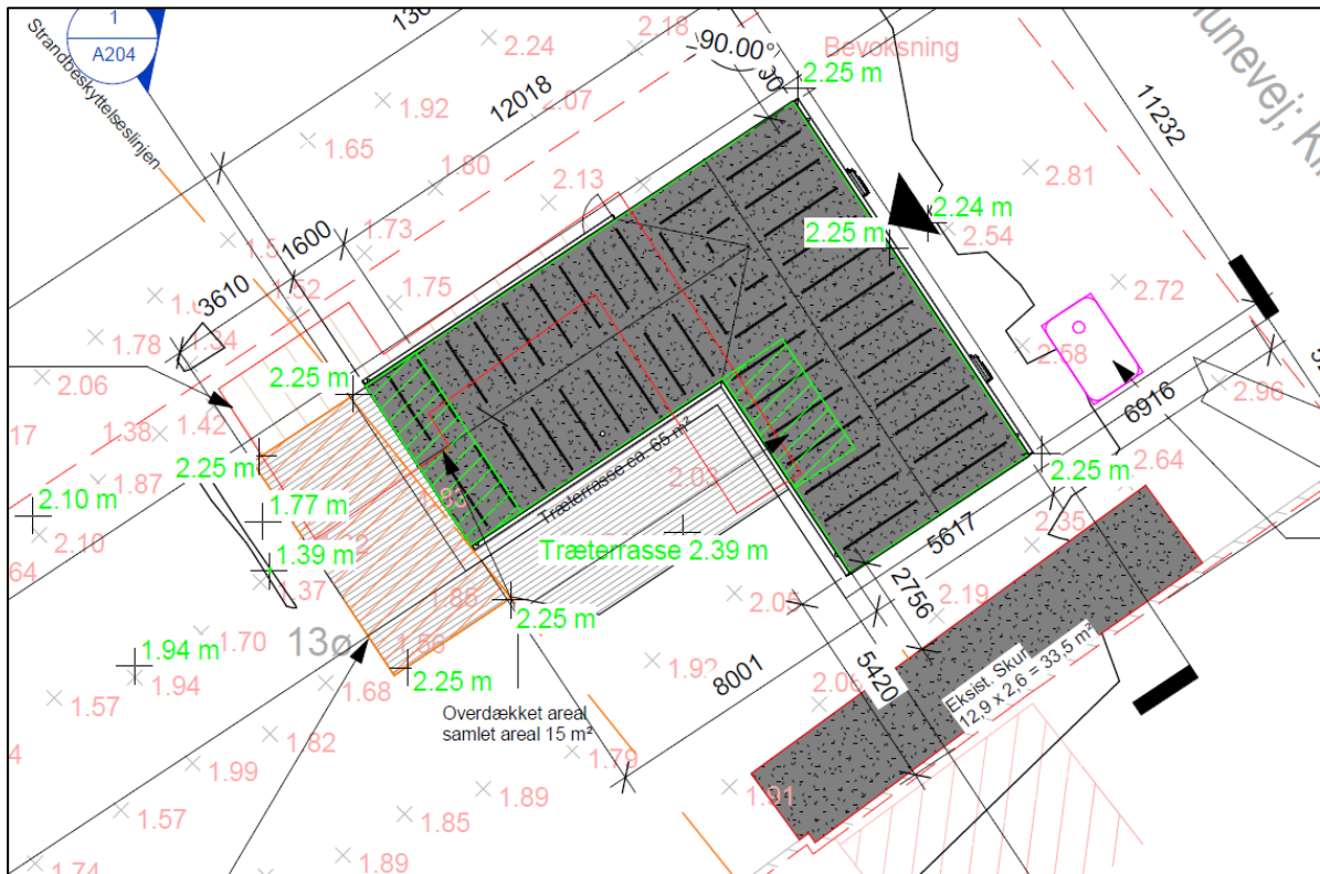
Situationsplan viser nyt sommerhus opført uden for strandbeskyttelseslinjen. Terrasse inden for strandbeskyttelseslinjen er vist med rød skravering.
