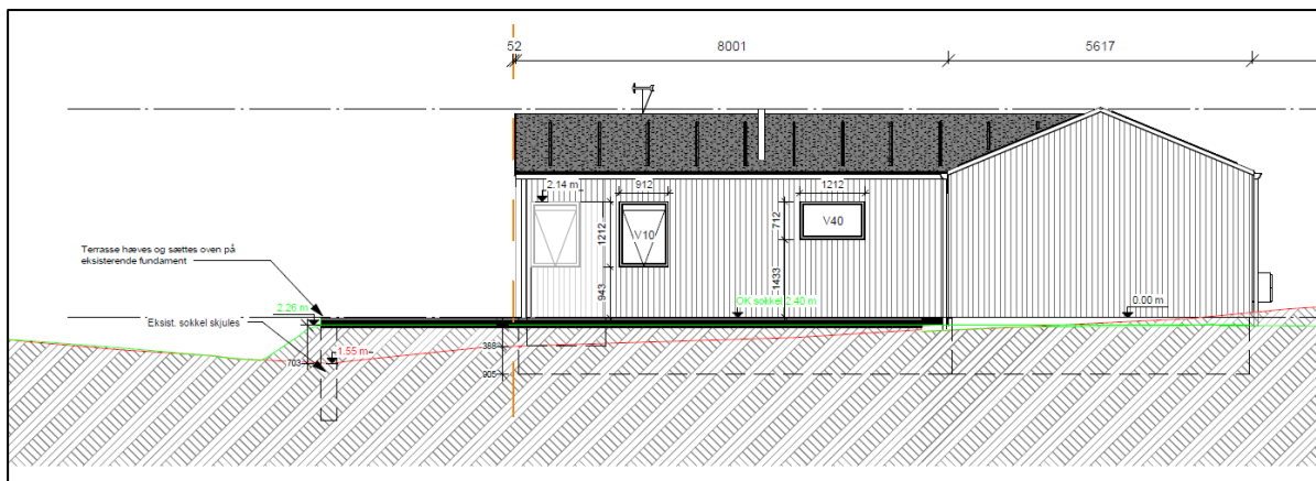
Snit viser nyt sommerhus fra sydøst. Den hævede terrasse ses til venstre på billedet. Terrænet fyldes op under terrassen for at skjule fundament fra eksisterende sommerhus.
