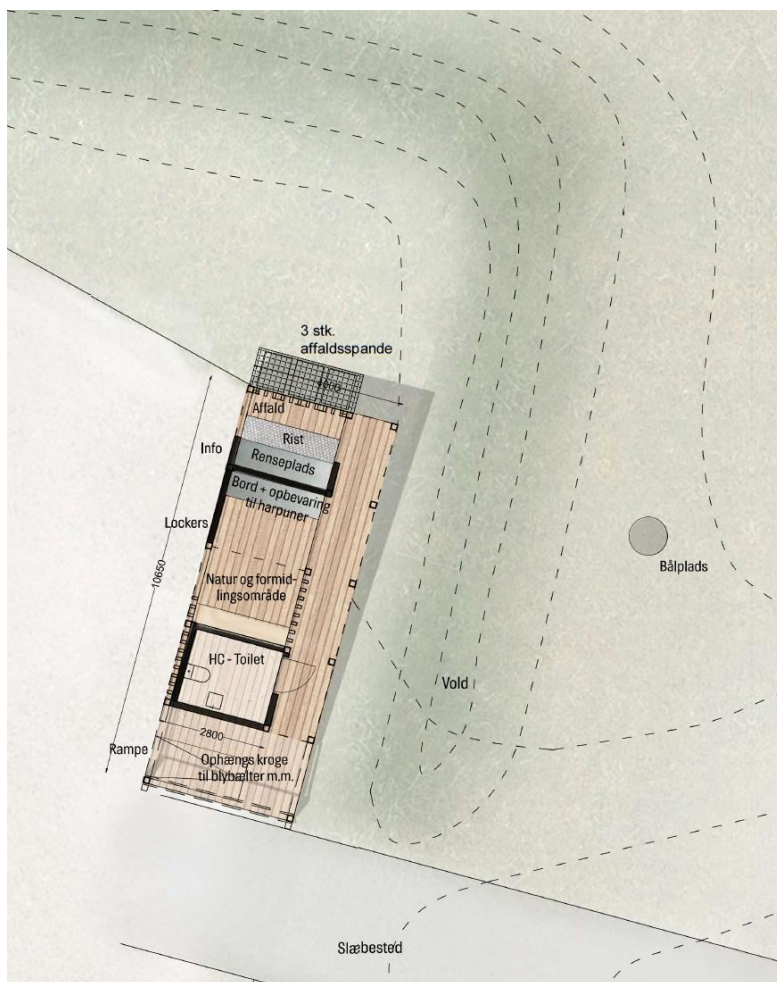
Fig. 6. Tilsendt fra ansøger. På figuren ses den ansøgte placering af affaldsbeholderne, der ligger nord for den ansøgte bygning.
