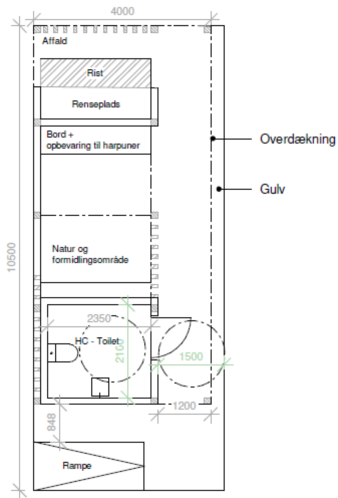
Fig. 3. Tilsendt fra ansøger. På figuren ses en plantegning over den ansøgte bygning.
