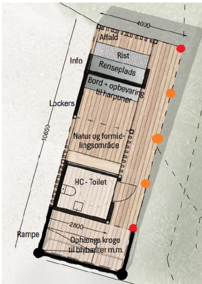
Fig. 4. Tilsendt fra ansøger. På figuren ses en tegning af den ansøgte formidlingsbygning. Søjler og bjælker markeret med sort fjernes. Søjler markeret med orange fjernes. Søjler markeret med rød bibeholdes.
