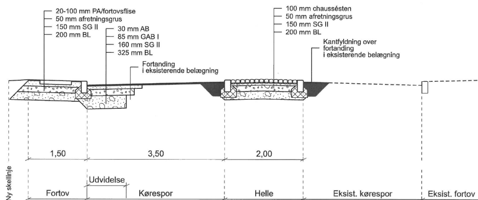
Tværsnit af udvidelse vej med nyt fortov
