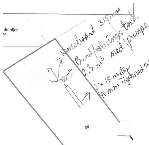
Anlæggets udformning
