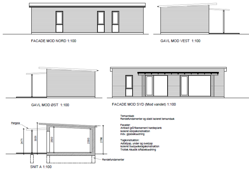
Fig. 3. Tegning til illustration af ønskede forhold.
