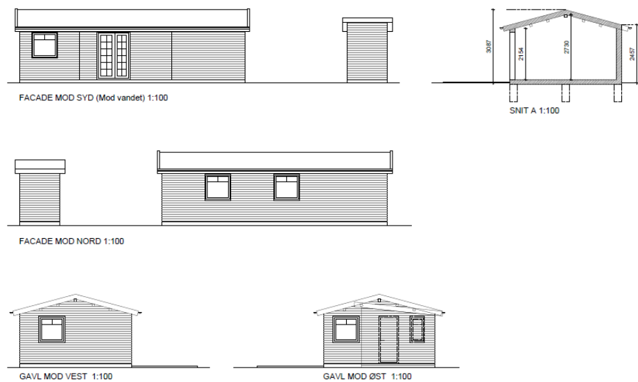
Fig. 2. Tegning til illustration af eksisterende forhold.
